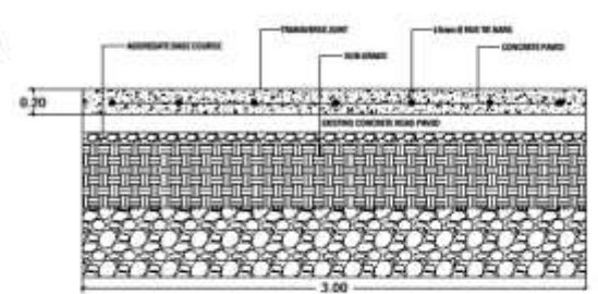
LONGITUDINAL CROSS SECTION - B SCALE: 1:50
