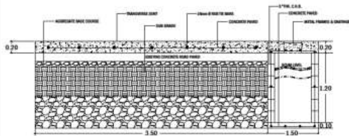
LONGITUDINAL CROSS SECTION - A SCALE: 1:50
