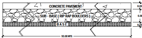
LONGITUDINAL SECTION - B SCALE: 1:80 MTS.
