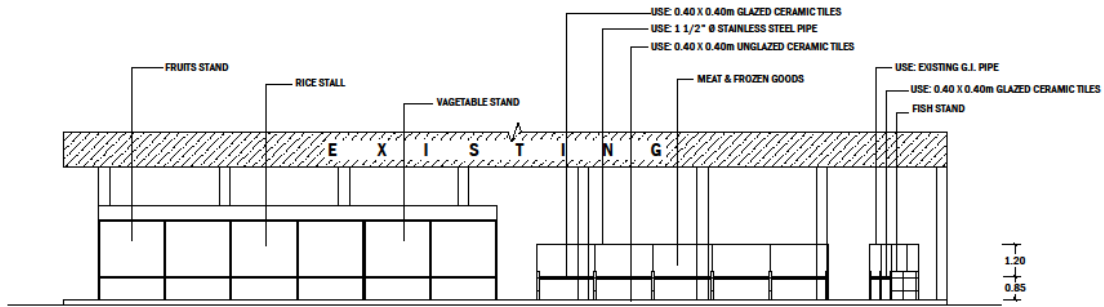
LATITUDINAL CROSS SECTION - B SCALE: 1:25 MTS.
