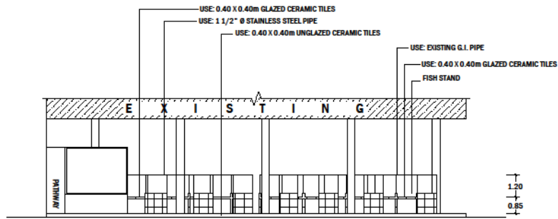
LONGITUDINAL CROSS SECTION - A SCALE: 1:25 MTS.
