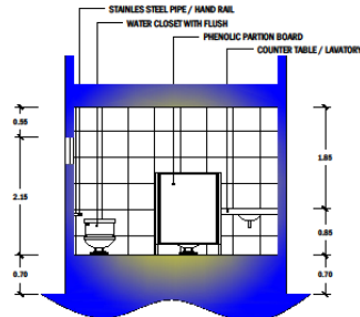
LATITUDINAL SECTION A - A
