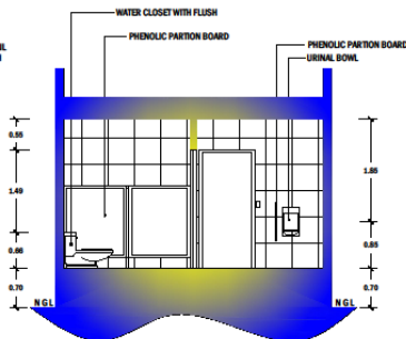
LONGITUDINAL SECTION D - D
