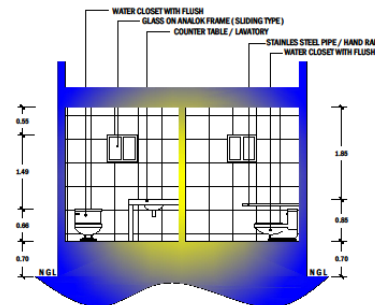
LONGITUDINAL SECTION C - C
