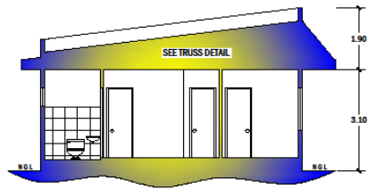
LONGITUDINAL CROSS SECTION - A SCALE: 1:450 MTS.
